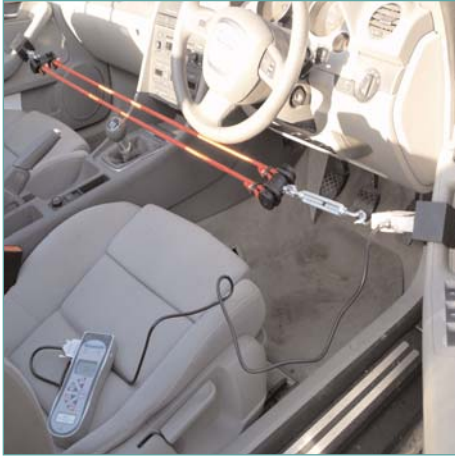
Door slam force test
